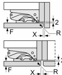
Masse in mm Empfehlung Spaltmasse für Flachscharnier
